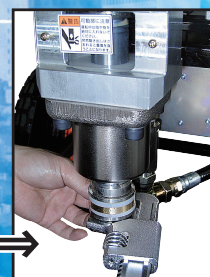
③ 吐出弁を外す。
